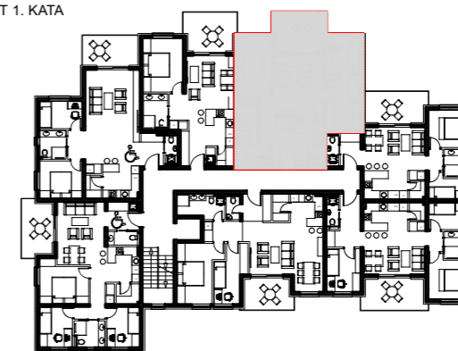
TLOCRT 1. KATA
