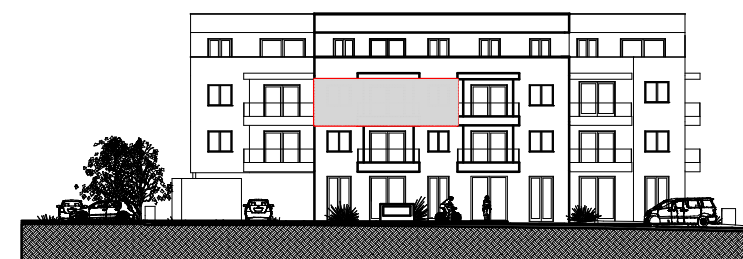
ZAPADNO PROČELJE
