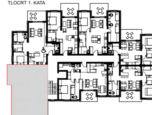
TLOCRT 1. KATA
